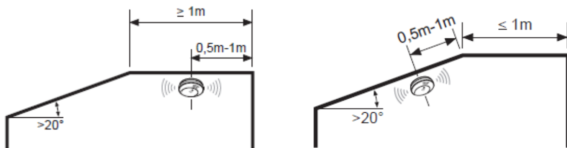
Abbildung 2: Befestigung des Rauchwarnmelders an der Decke
